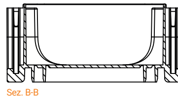
Sez. B-B
