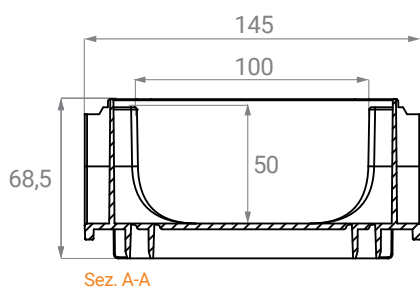
Sez. A-A
